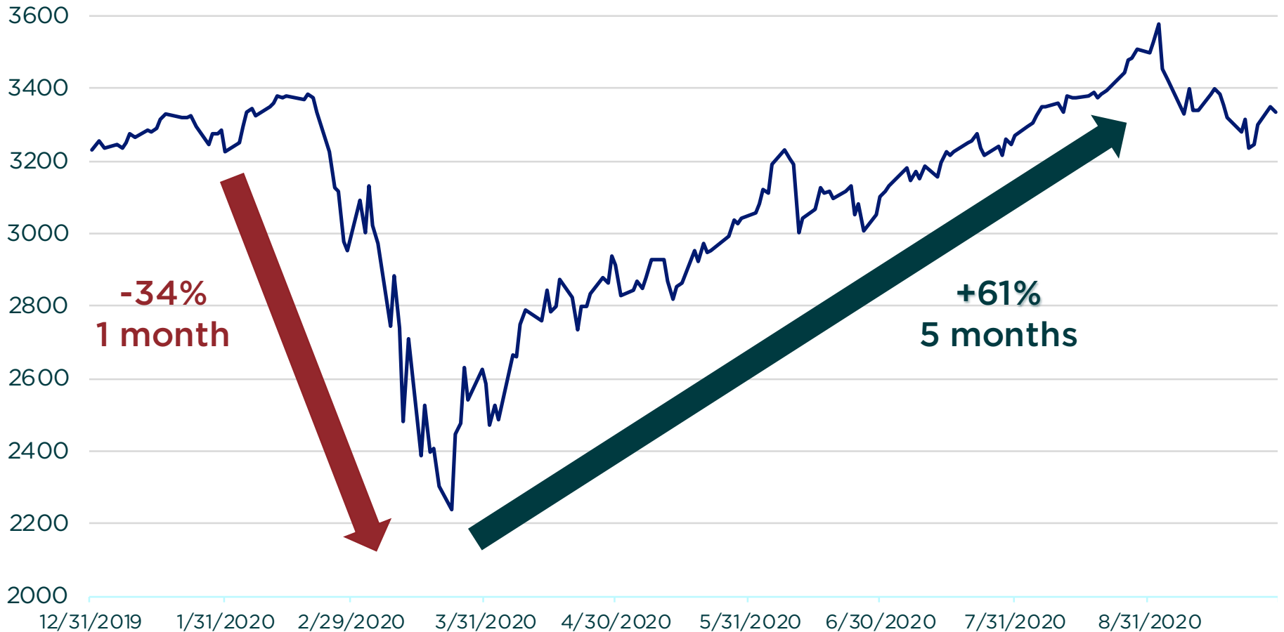
S&P 500
